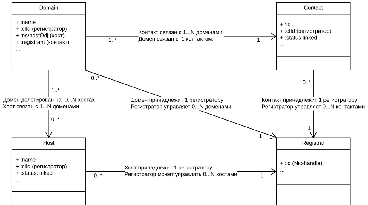
Рис. 2. Диаграмма связей объектов реестра
